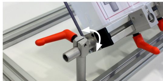
Schwenkvorrichtung
